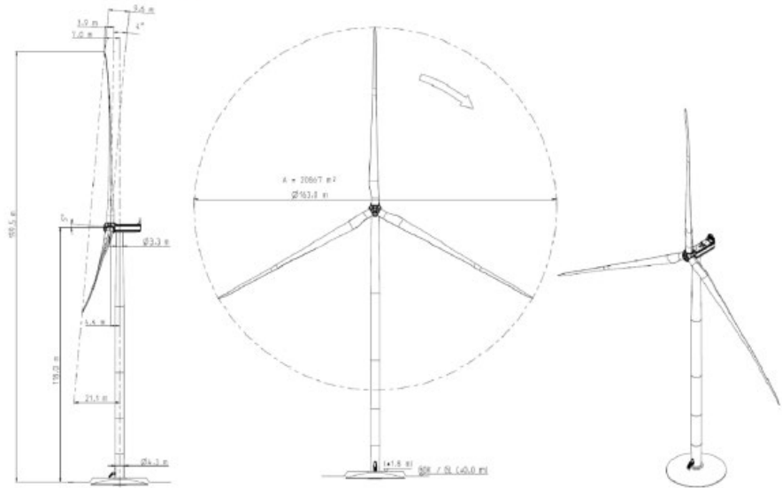
Figura 4. Detalle del aerogenerador seleccionado
